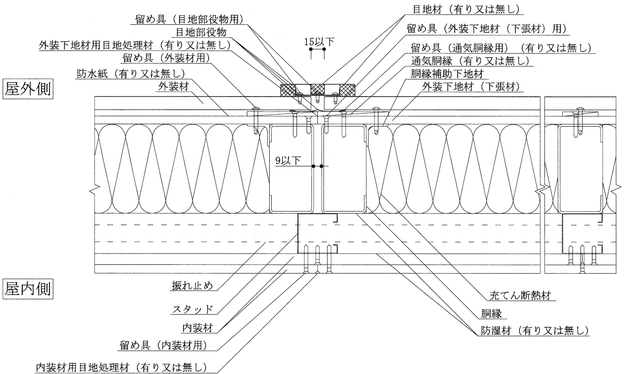
水平断面詳細図
