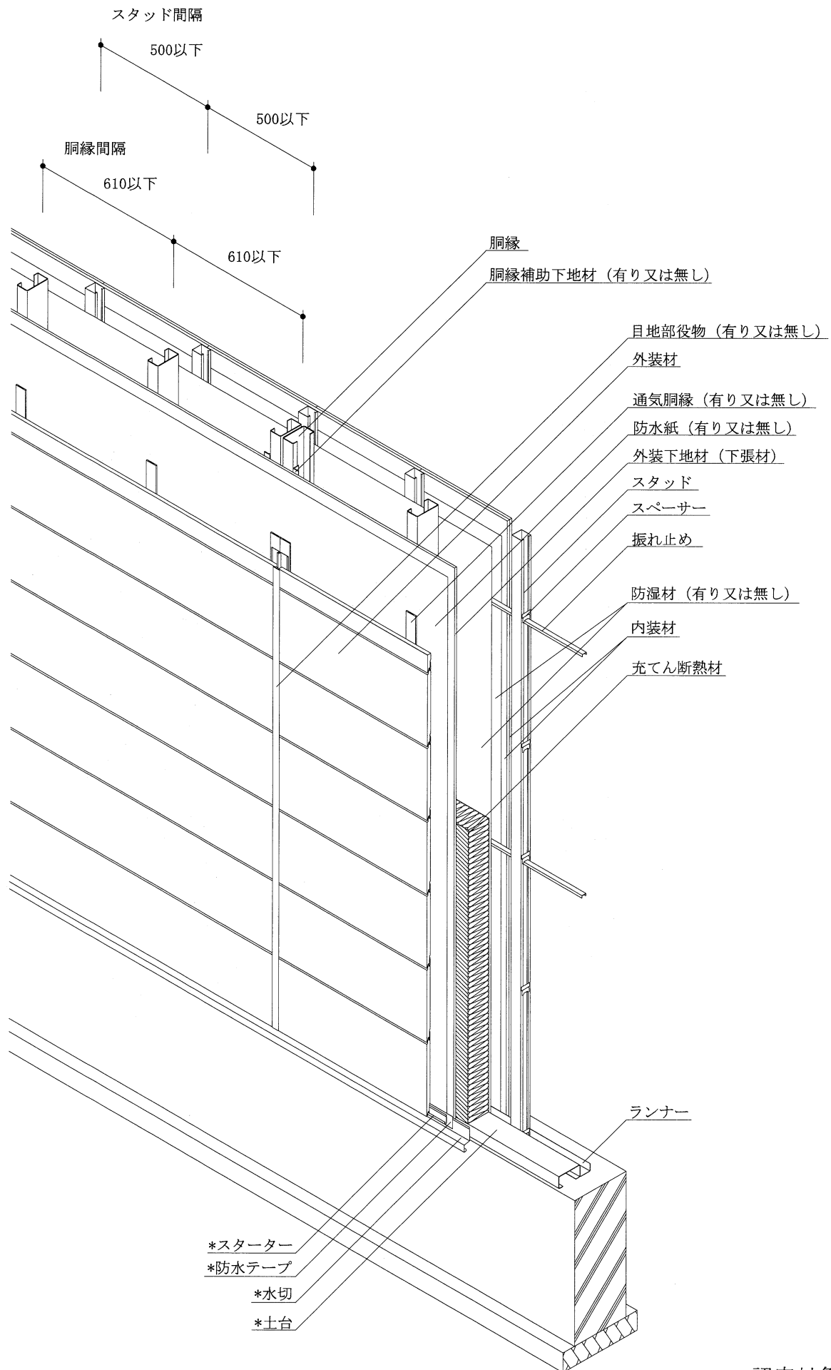
透視図 (別添-14)
